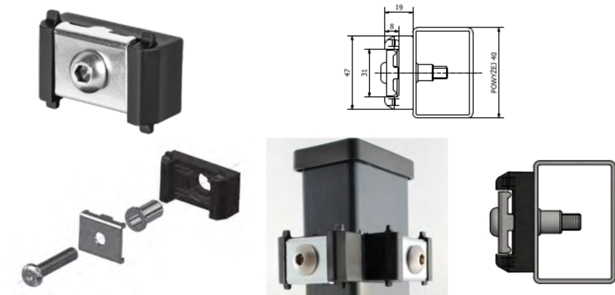
ŚRUBA M8x40
